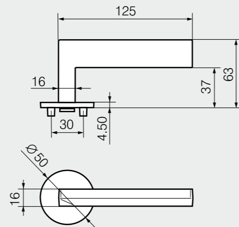
Технический чертёж
